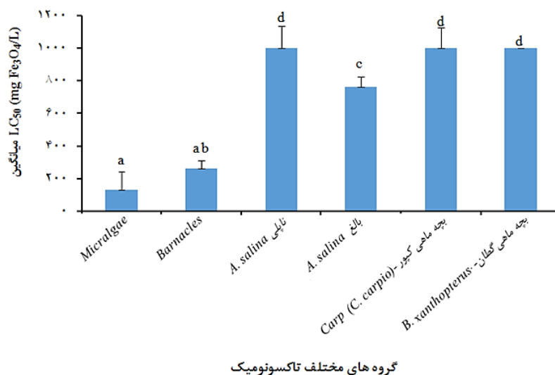
شکل ۲ - اختلاف میانگین L(E)C_{50} حساسیت گونه‌ای سطوح مختلف تاکسونومیک زنجیره‌های غذایی زیست بوم دریایی در مواجهه حاد با نانوذرات مگنتیت شیمیایی ( Fe_3O_4 ).
