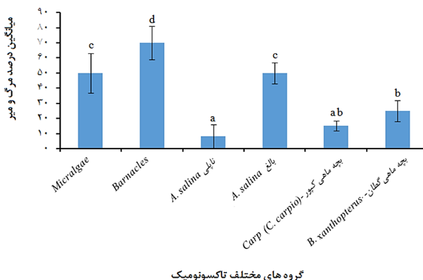
شکل ۳ - میانگین درصد مرگ و میر گونه‌ای در سطوح مختلف تاکسونومیک زنجیره‌های غذایی زیست بوم دریایی در مواجهه حاد با نانوذرات مگنتیت شیمیایی ( Fe_3O_4 ).
